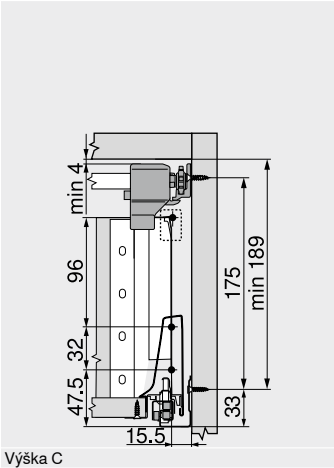
Výška C
