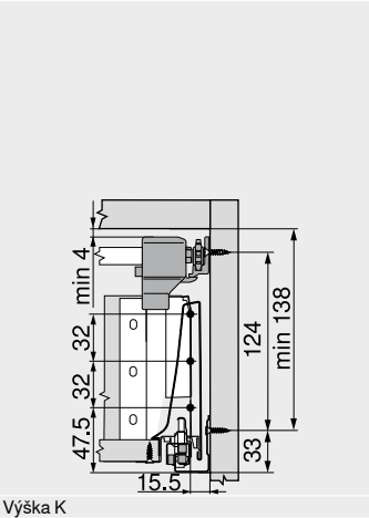
Výška K
