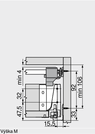
Výška M
