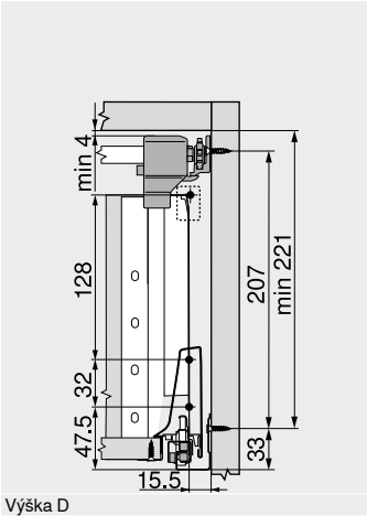
Výška D
